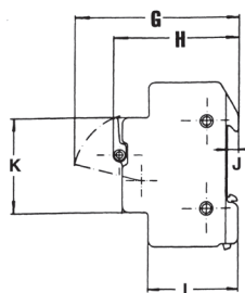
Tiges d'attache USPTH
